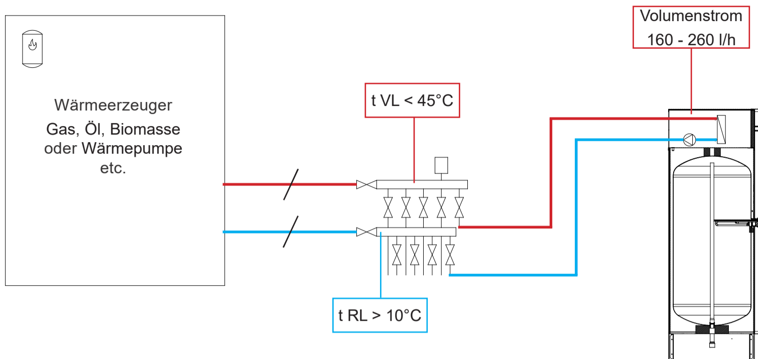
Schema 1 Anschluss über FBH Verteiler - Vorlauf
